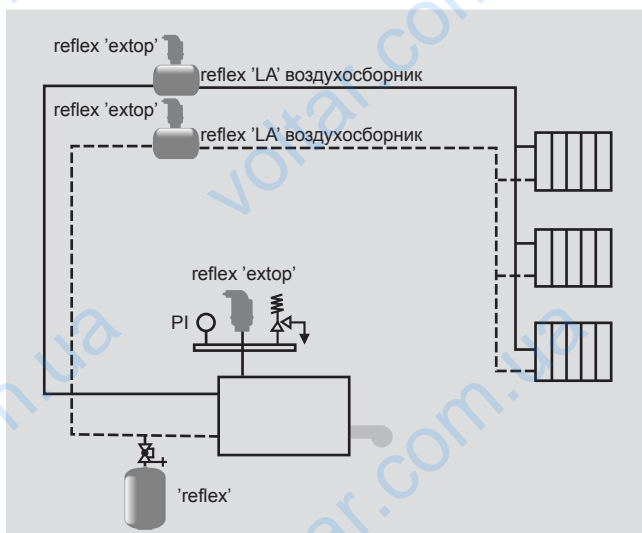
reflex 'extop' и воздухооборник в системе после её заполнения
