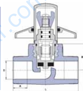
Вентиль проходной "lux" с хромированным кожухом под штукатурку
