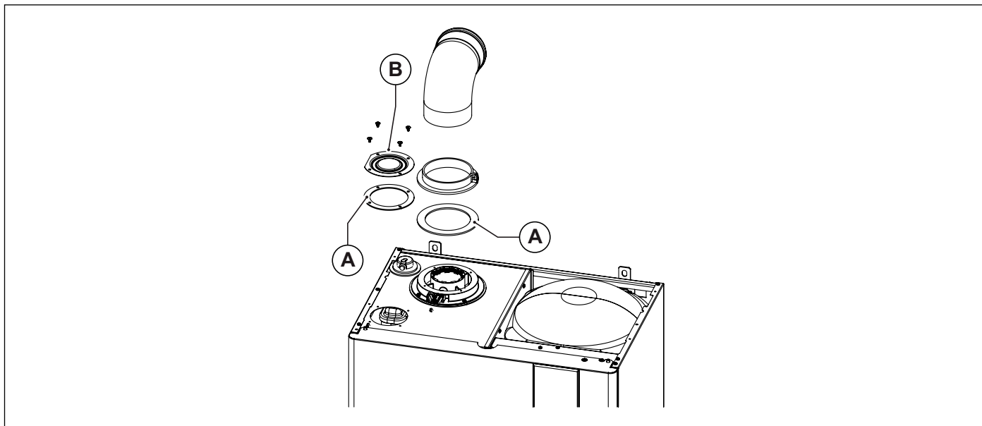
Рис. 9 Коаксіальні дымоходи типу C13 - C33
