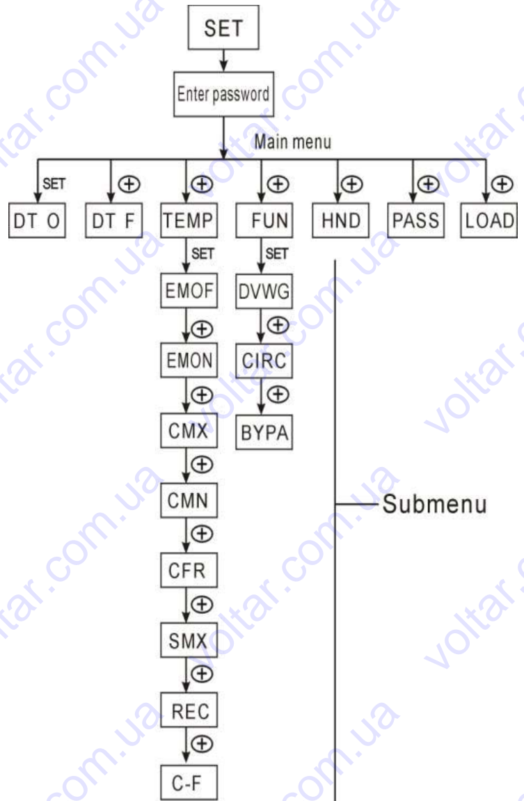
Меню контроллера SR868C9
