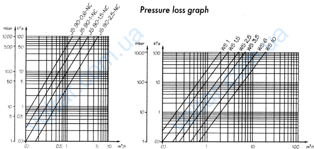
Таблиця 10.2. Технічні характеристики і графіки втрати тиску для витратомірів JS, WS
