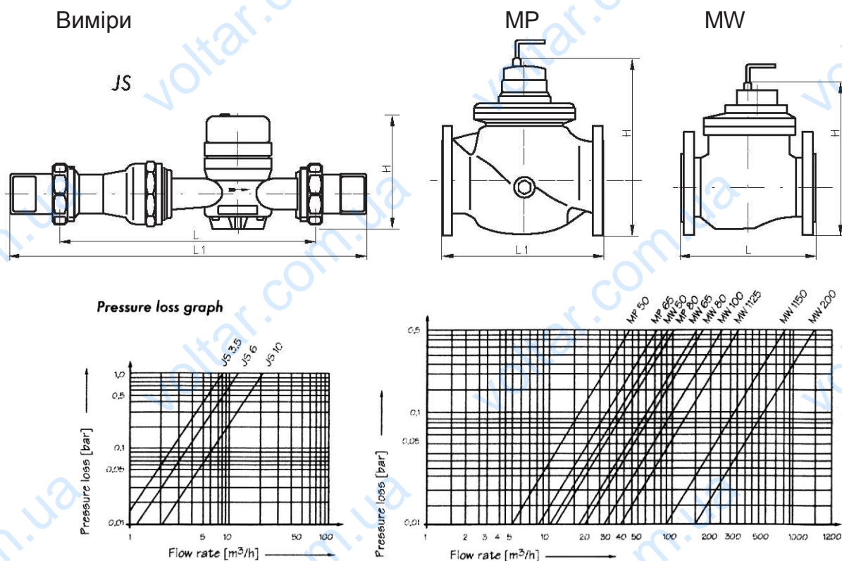
Рис. 10.1. Графіки втрати тиску для витратомірів JS, MP, MW
