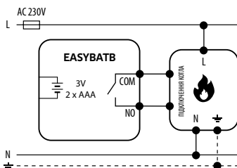
а) Схема підключення до котла
