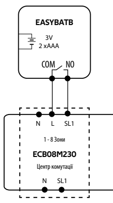
в) Схема підключення до центру комутації
