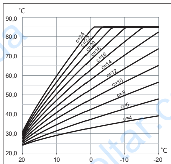
Кoeffициент наклона кривой нагрева
