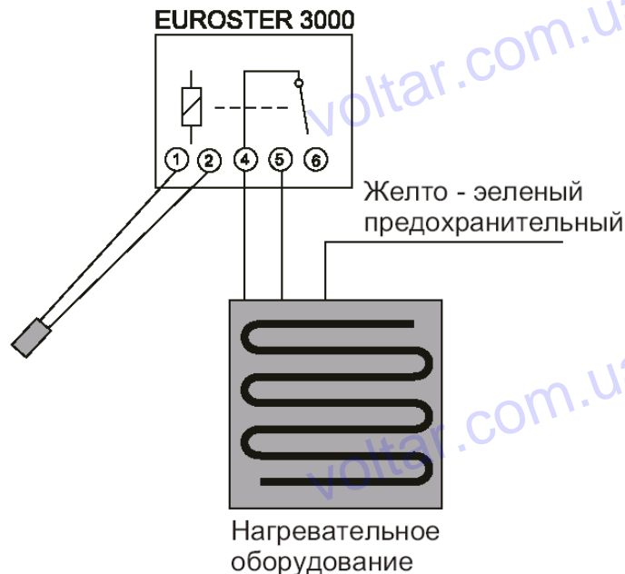
Половой датчик
