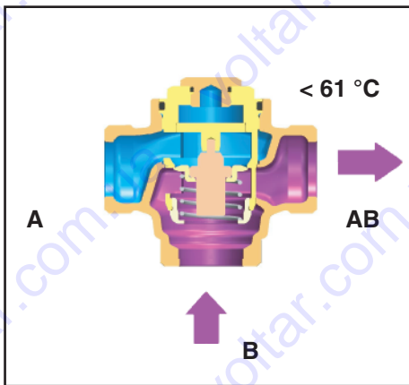
Клапан закрыт (Положение при пуске)
