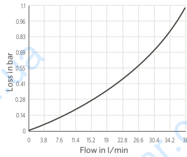
ПОТЕРИ НА ТРЕНИЕ ПОДВИЖНЫХ СОЕДИНЕНИЙ
