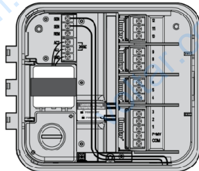
Провода датчика к клеммам SEN
