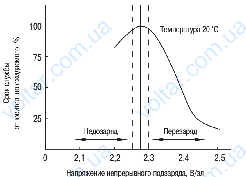
Рис. 13 Зависимость срока службы аккумулятора от напряжения подзаряда.
