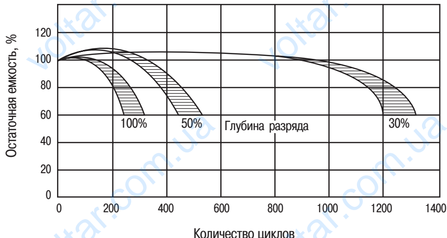
Рис. 11 Зависимость количества циклов от глубины разряда аккумуляторов Ventura.
