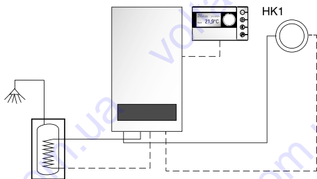
Комплектация одноконтурного котла с погодозависимым управлением контуром отопления и системой горячего водоснабжения (вертикальный бак-водонагреватель SU, для монтажа рядом с котлом)
