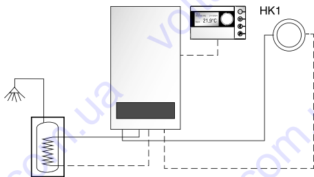
Комплектация одноконтурного котла с погодозависимым управлением контура отопления и баком косвенного нагрева
