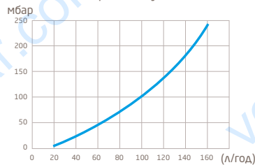
Втрати тиску SB25+V
