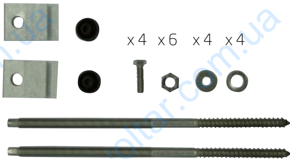
LNC 71027003 Комплект кріплень на скатний дах SVB 26
