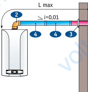
Коаксіальний димар з горизонтальним виводом через стіну
