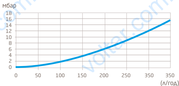
Втрати тиску SVB26
