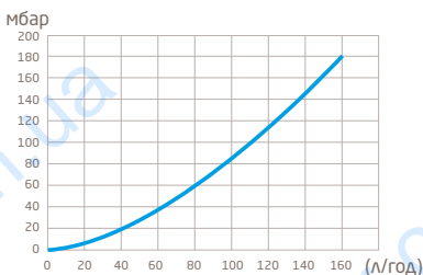
Втрати тиску SB20+0
