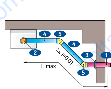
Коаксіальний димар з горизонтальним виводом через стіну
