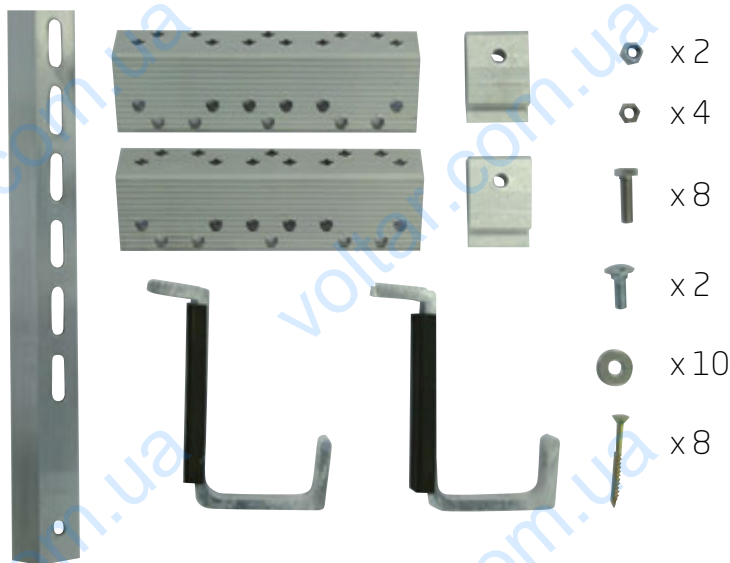
LNC 71027006 Комплект кріплень на скатний дах SVB 26 - вертикальна орієнтація
