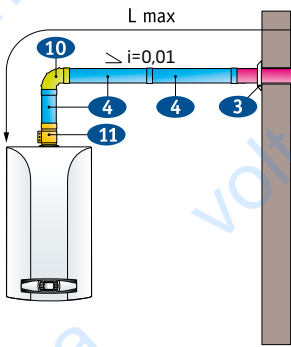
Коаксіальний димар з горизонтальним виводом через стіну
