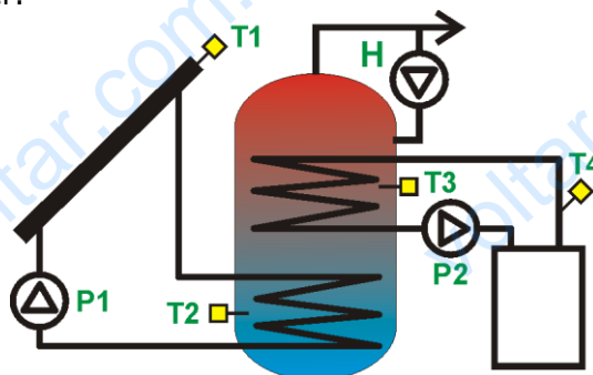
Fig. 13.7 Solar thermal scheme G
