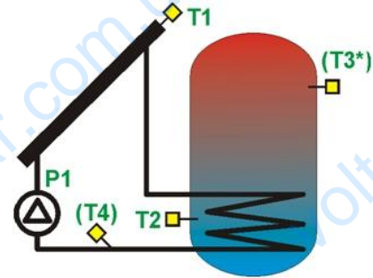
Fig. 13.1 Solar thermal scheme A
