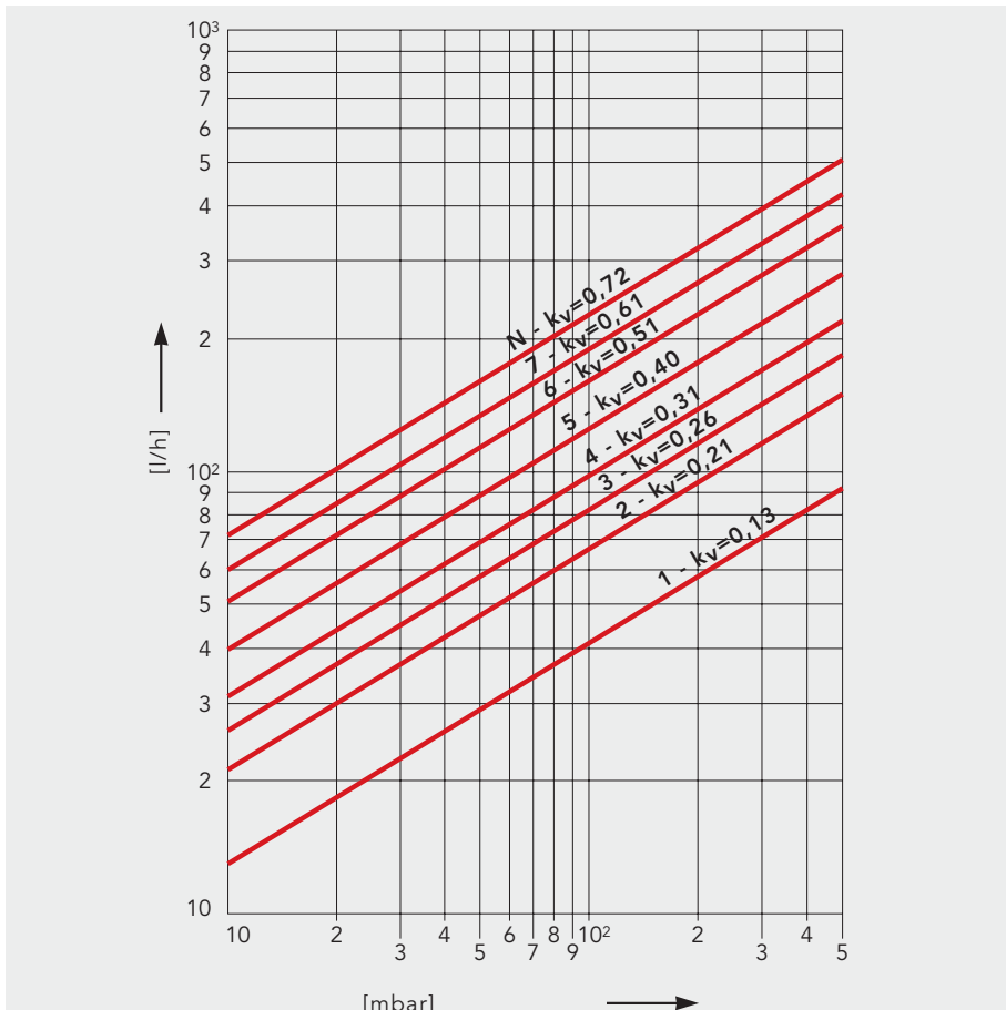
Диаграмма 1 Потеря давление [мбар] - двухтрубная система при пропорциональном отклонении 2K
