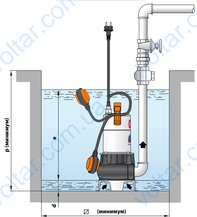
Типовая схема монтажа
