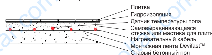
Новый пол поверх старого бетонного - влажные помещения
