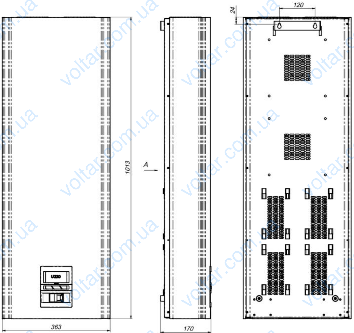
Рисунок 10. Установчі та посадочні розміри стабілізаторів Герц і Герц-Дуо на 100-125А
