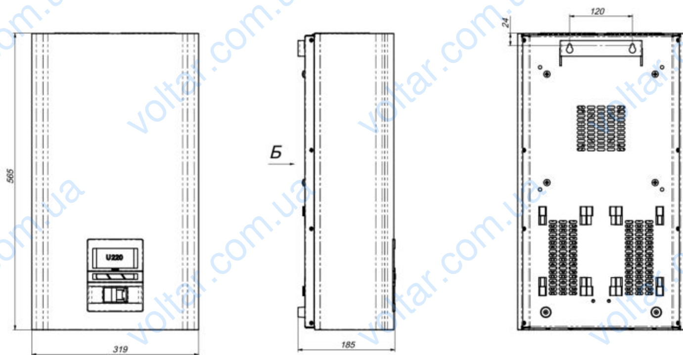
Рисунок 9. Установочные и посадочные размеры стабилизаторов Герц и Герц-Дуо на 80 А
