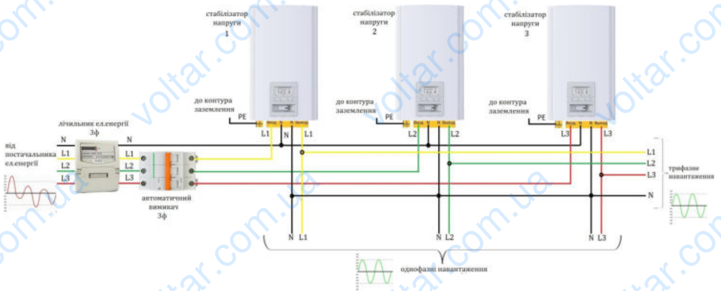
Рисунок 12. Схема підключення стабілізатора до трифазної мережі
