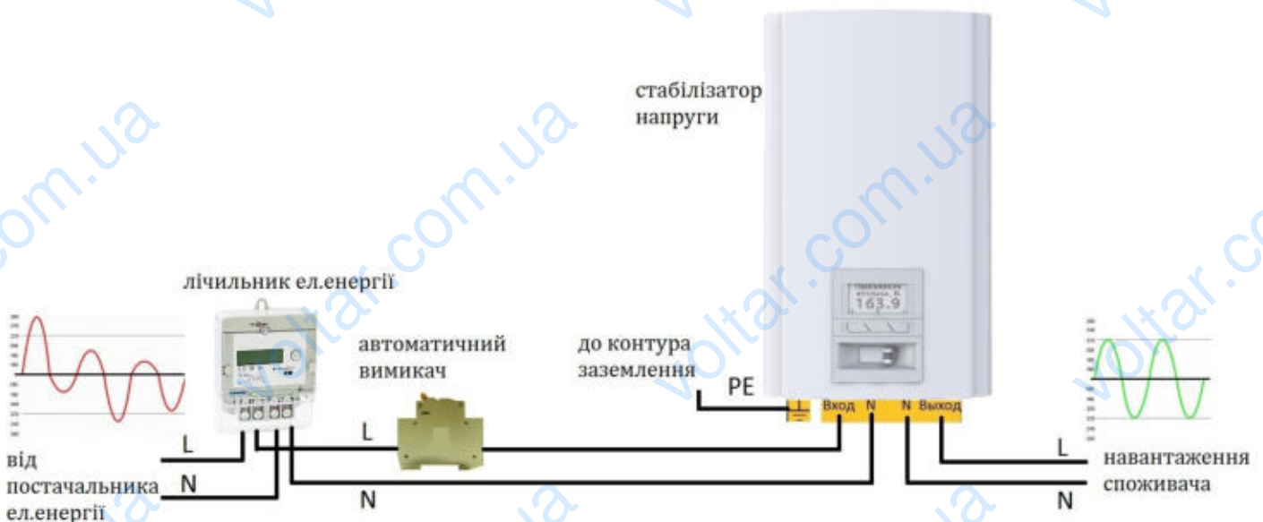
Рисунок 11. Схема підключення стабілізатора Герц і Герц-Дуо до однофазної мережі
