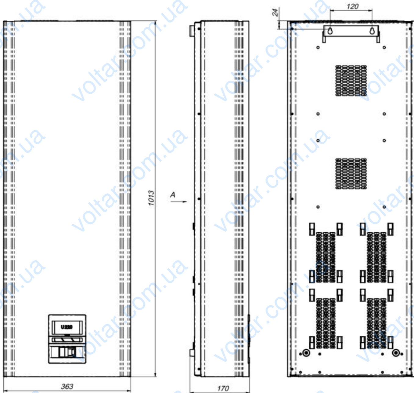
Рисунок 10. Установочные и посадочные размеры стабилизаторов Герц и на 100-125 А
