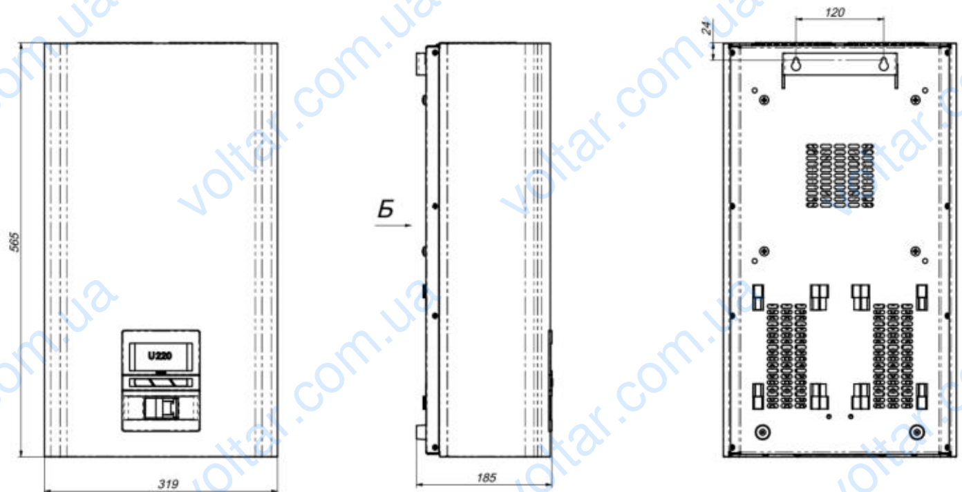
Рисунок 9. Установчі та посадочні розміри стабілізаторів Герц і Герц-Дуо на 80А
