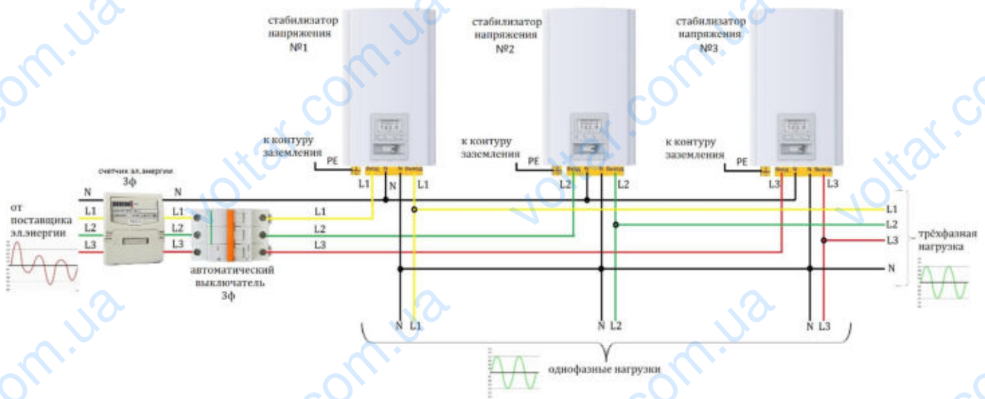
Рисунок 12. Схема подключения Герц и Герц-Дуо к трёхфазной сети
