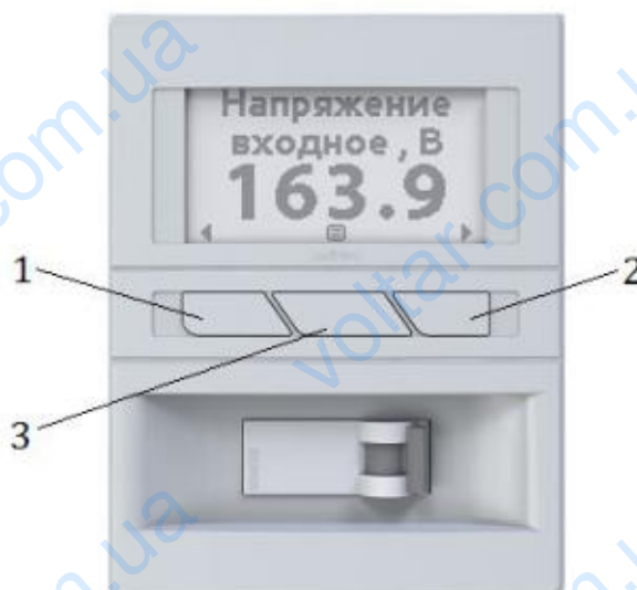
Рисунок 14. Расположение кнопок управления на панели управления Герц V3.0
