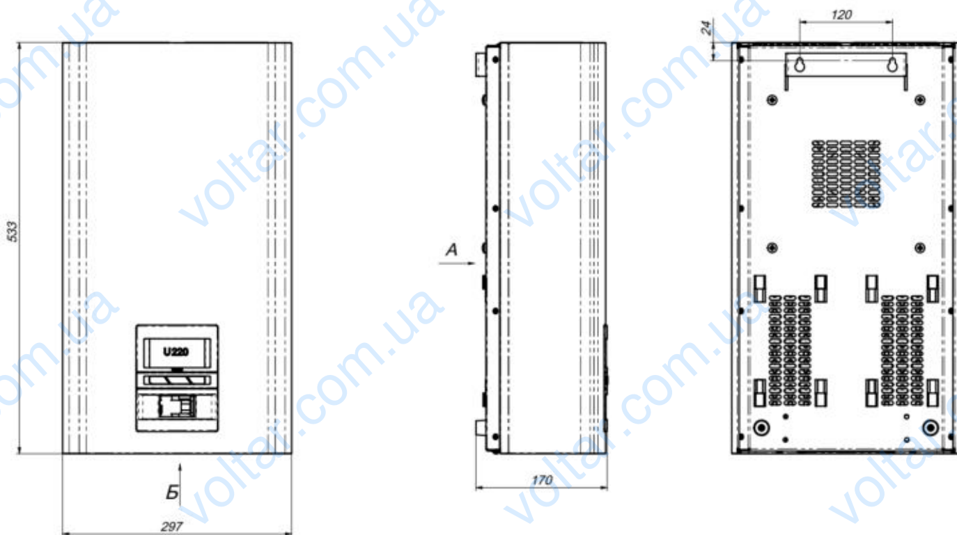
Рисунок 8. Установочные и посадочные размеры стабилизаторов Герц и Герц-Дуо на 50-63 А
