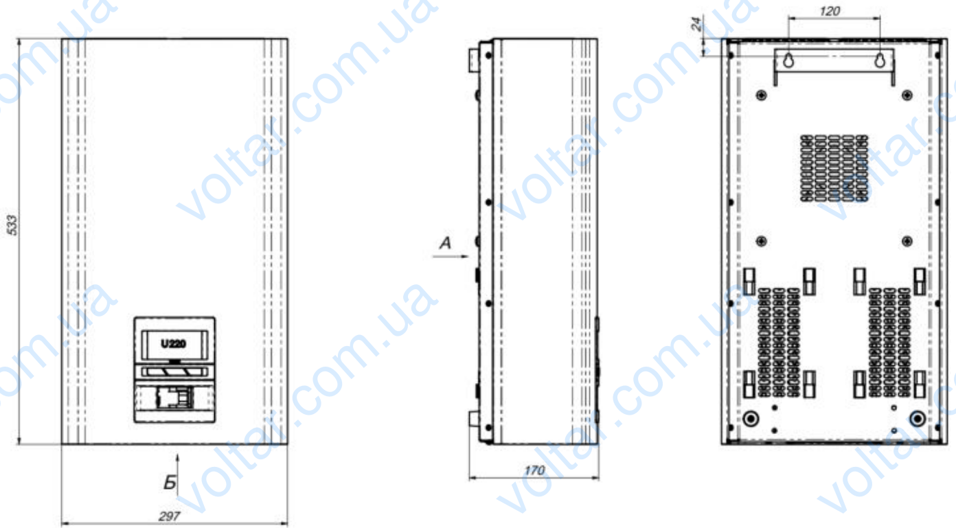
Рисунок 8. Установчі та посадочні розміри стабілізаторів Герц і Герц-Дуо на 50-63А
