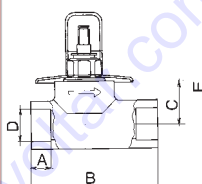
Вентиль Laguna под штукатурку с пласт. колпаком
