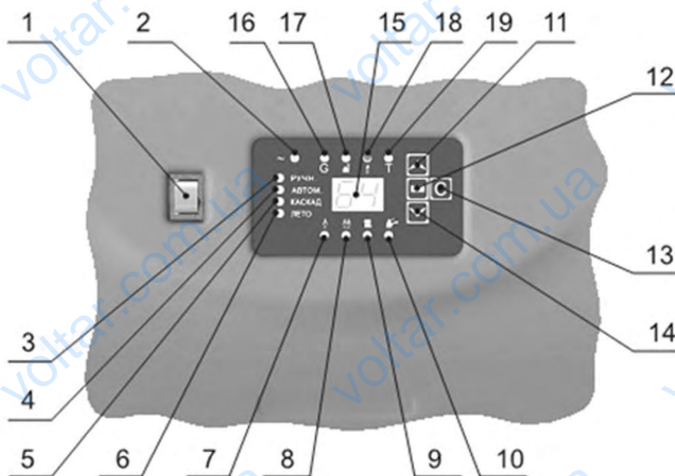
Рис. 2 Пульт управления с котловым контроллером котла «Smart», «Smart SL/SR»
