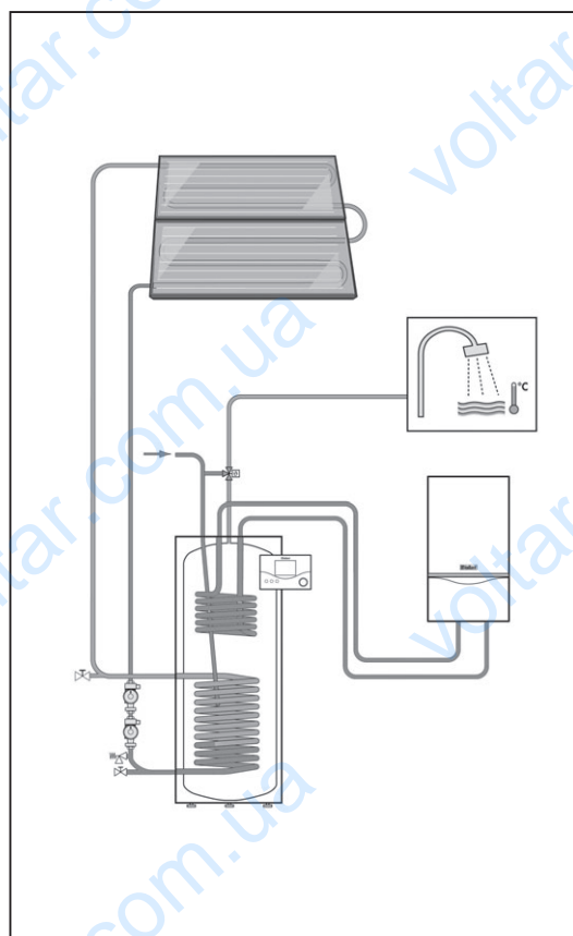
Солнечная система auroSTEP plus 2.250 P
