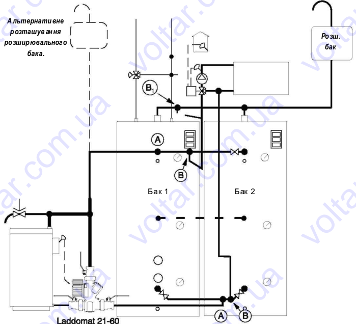
Laddomat 21-60
