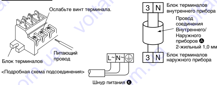
Шнур питания
