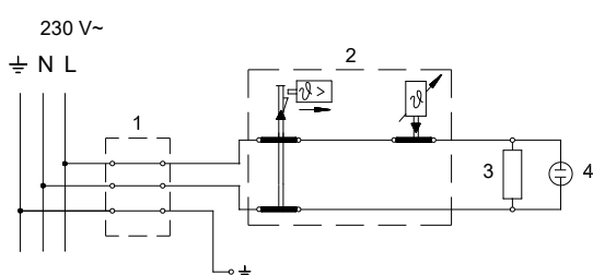
Электросхема
