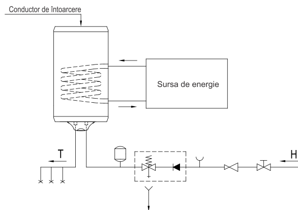
Sistemul închis (sub presiune)
