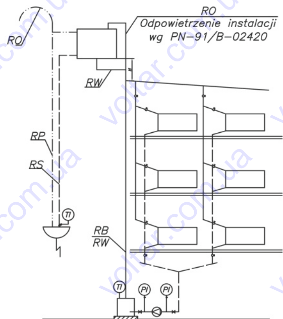
Рис.6. Примерная схема защиты водной системы центрального отопления, состоящей из одного котла или теплообменник, верхней часть, насос установлен на возврате
