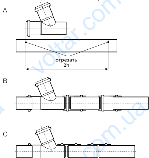
Рис. 14 Установка дополнительного тройника
