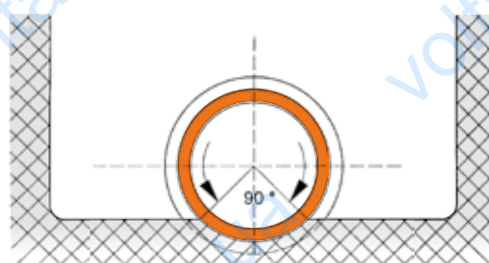
Рис. 5 Укладка в ненарушенный грунт естественного залегания (тип основы 2)
