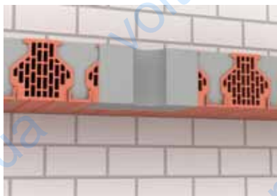
Перекрытия с ребристыми или кирпичными элементами
