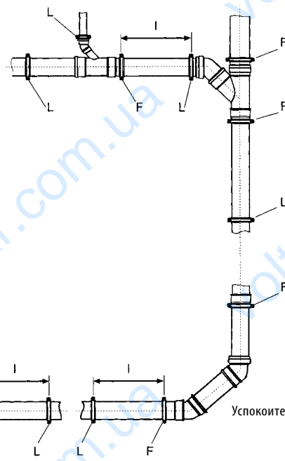
Хомут с прокладкой как плавающее крепление
