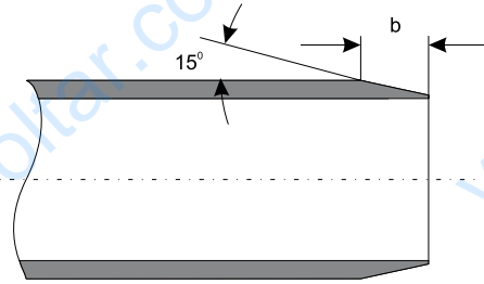
Рис. 3а Скос на конце трубы
