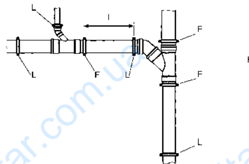
Хомут с прокладкой как плавающее крепление
