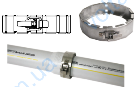
SK – Страховочный хомут (для ливневой канализации, 2,0 Бар)*
