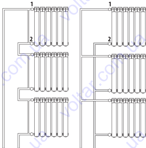
Однотрубная система с байпасами
