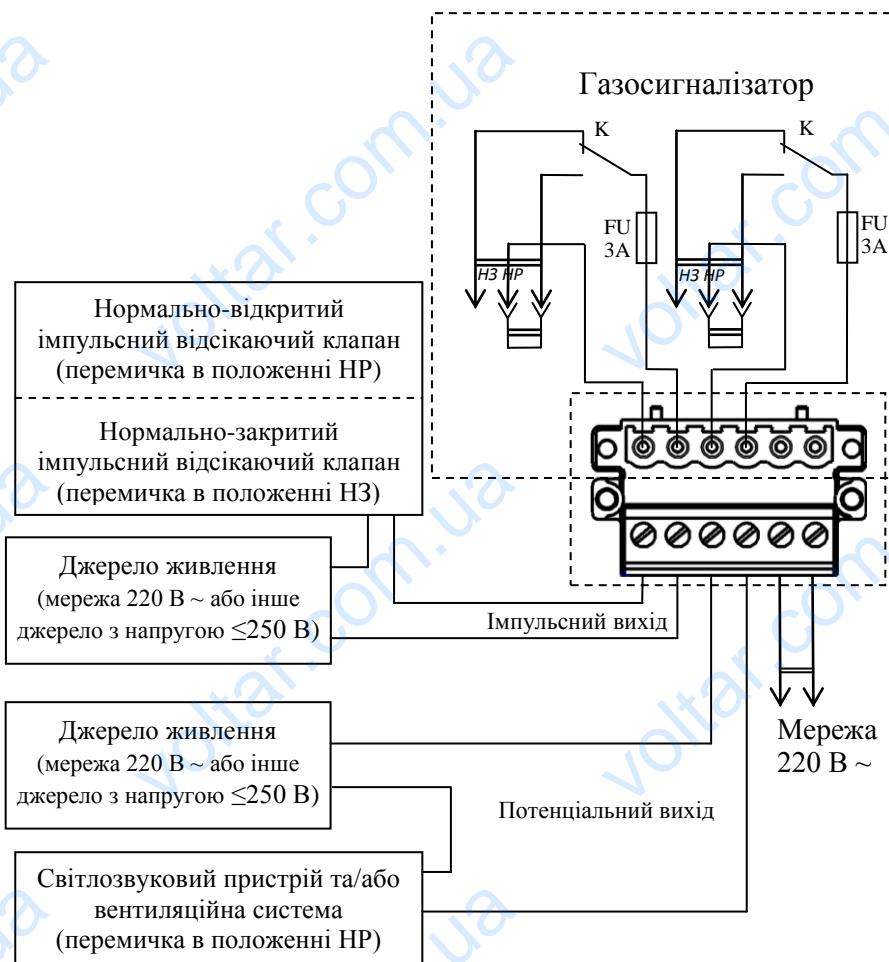
Рисунок 3. Схема підключення газосигналізатора «Страж SxxA2xE» (тобто, з типом управляючих виходів № 2 та настінним роз'ємом) до нормально-відкритого імпульсного відсікаючого електромагнітного клапану (типу EVG/NA, EVRM-NA, M16/RM-NA та ін.), світлозвукового пристрою, нормально-закритого електромагнітного клапану з потенціальним або імпульсним керуванням.
