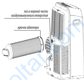
Прикрепление воздуховода к кондиционеру
